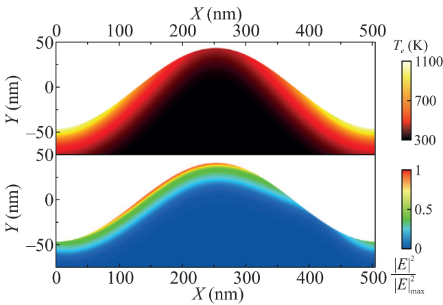
Рис. 2. (Цветной онлайн) Верхняя панель: рассчитанное в рамках двухтемпературной модели распределение электронных температур на одном периоде образца спустя \tau = 500 фс после прихода импульса накачки (800 нм). Нижняя панель: распределение квадрата электрической компоненты ближнего поля зондирующего импульса в образце на длине волны возбуждения поверхностного плазмона (617 нм), нормированное на максимум
